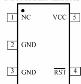
PT7M62xxCLXTA5 PT7M62xxNLXTA5
