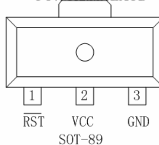
PT7M62xxCLXTD PT7M62xxNLXTD
