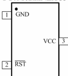
PT7M62xxCLXC3 PT7M62xxNLXC3
