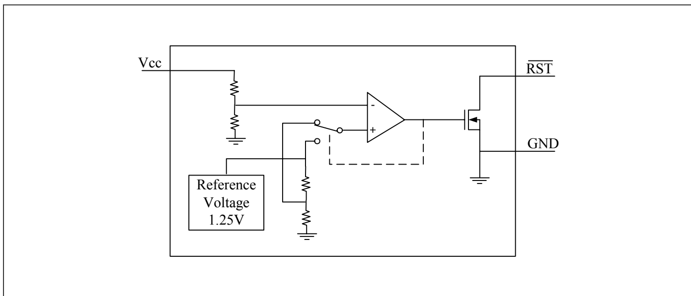
Block Diagram of PT7M62xxNL/NLL
