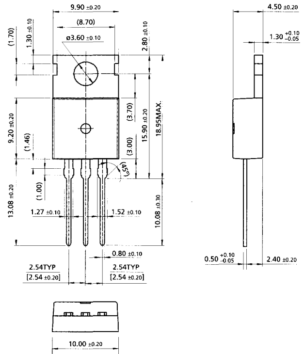
TO-220 (FS PKG Code AE)
