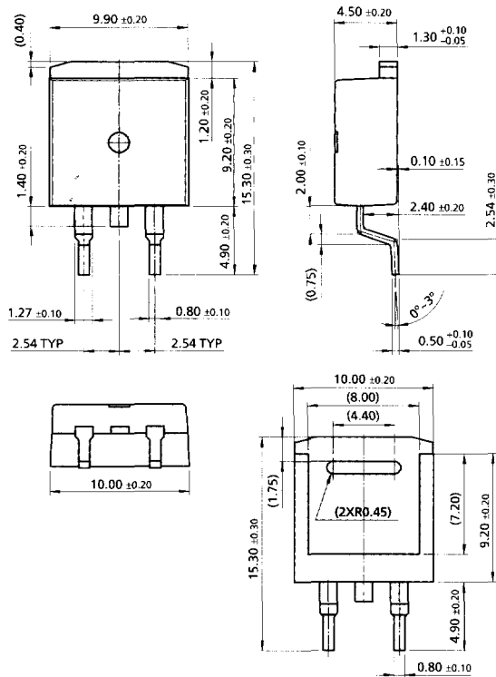
D 2 -PAK (FS PKG Code AB)
