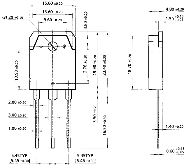
TO-3P (FS PKG Code AF)
