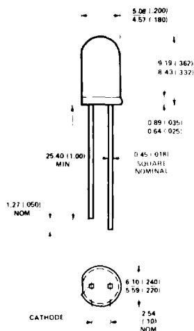
HLMP-4700, -4719, -4740
