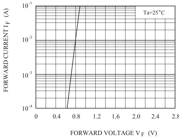
I_F - V_F
