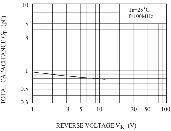
C_T - V_R
