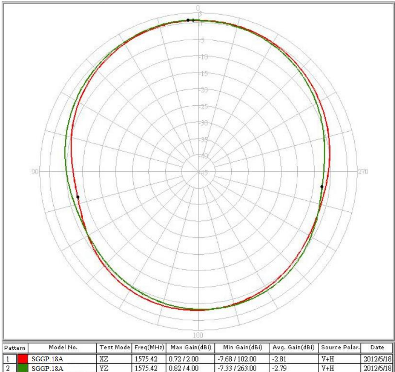
1575.4 MHz XZ+YZ-Plane
