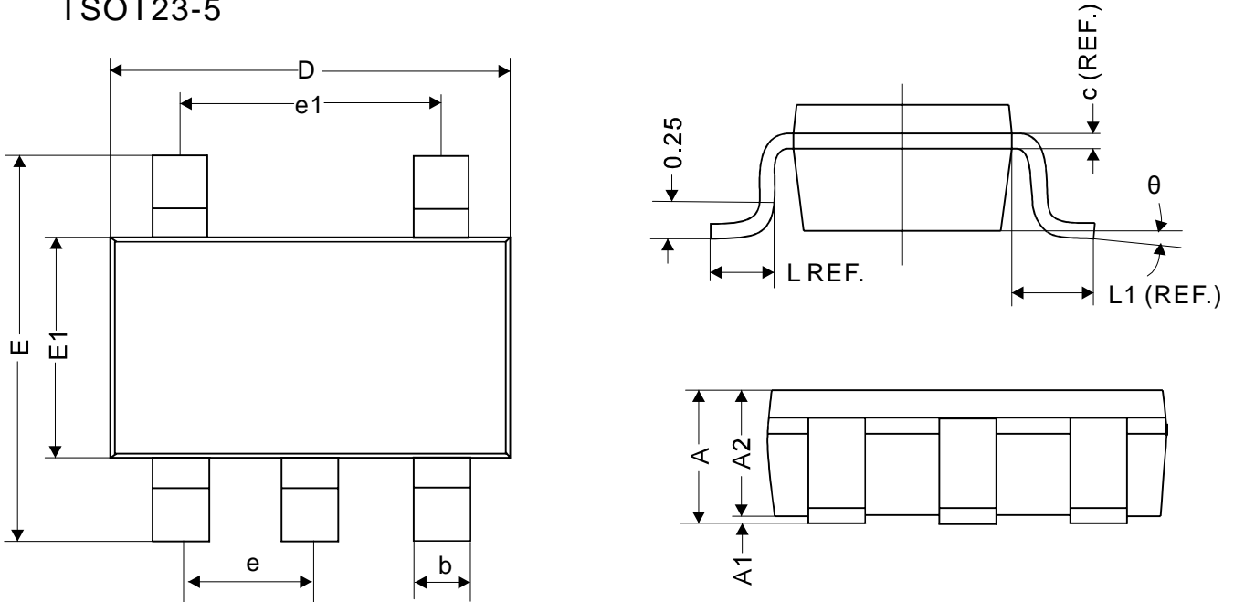
TSOT23-5
