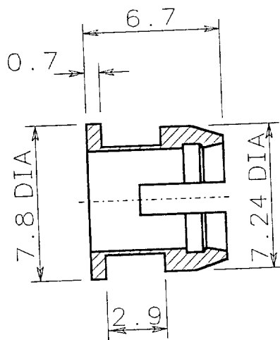
Clip
