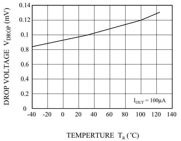
Fig. 4 T_a - V_{DROP}
