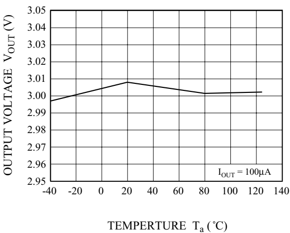
Fig. 5 T_a - V_{OUT}
