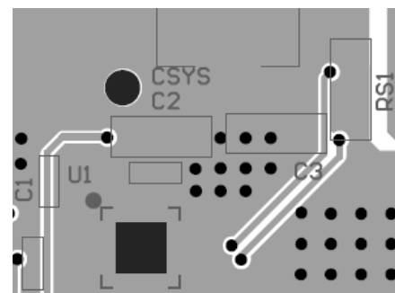
Bottom Layer
