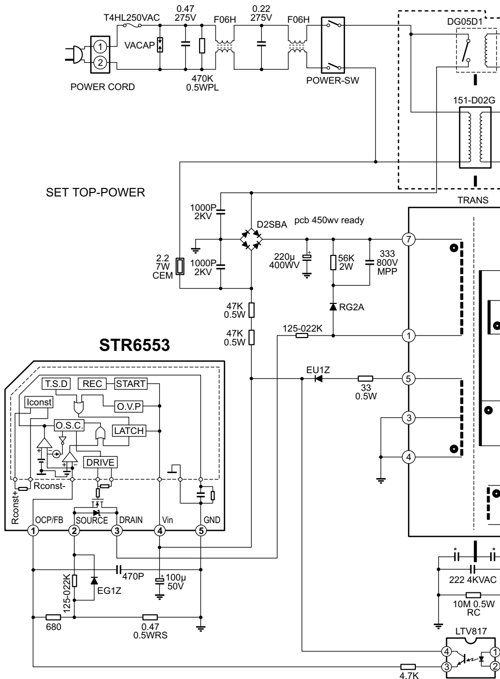
Rys.1. Aplikacja układu STR6553 w OTVC MZ40PA10 firmy LG.
