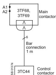
3TF6. 33-Q..
