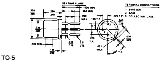
TO-5
