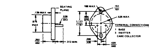
TO-3
