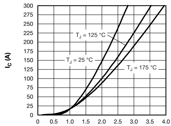
93185_02 V_{CE} (V)
