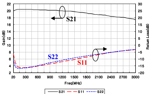
S-parameter
