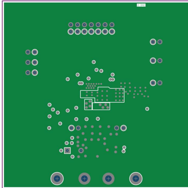
Copper Layer 2
