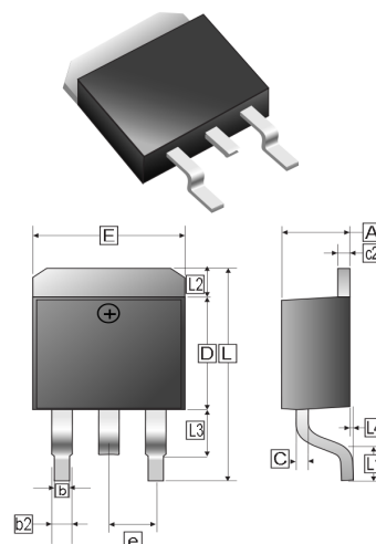
TO-263
