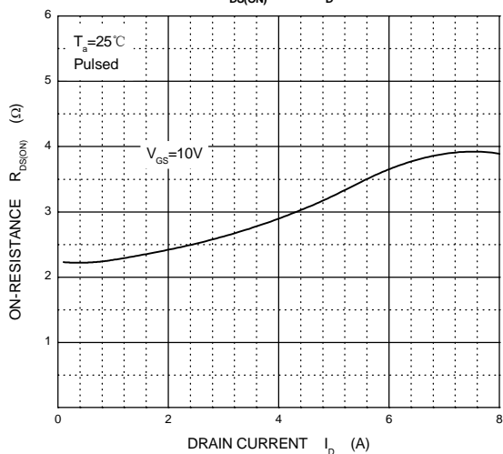
R_{DS(ON)} — I_D
