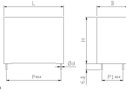
BOX Style: 4 Wires
