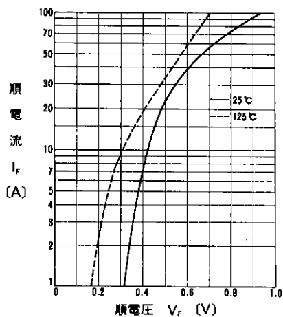
順特性
