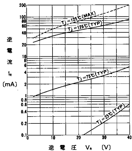
逆特性
