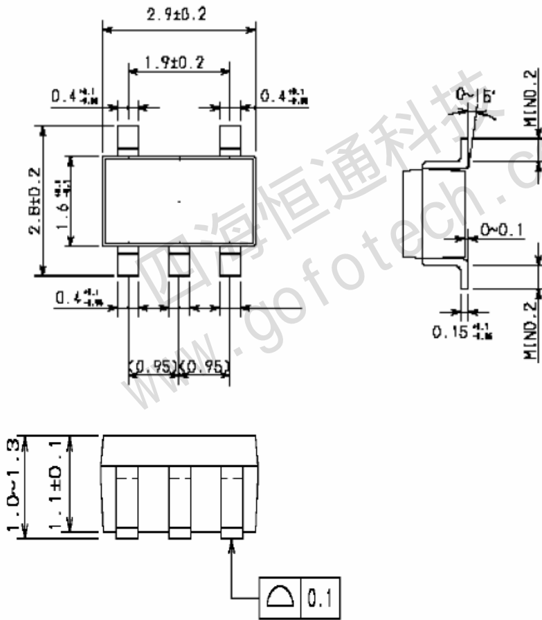
SOT-23-5L
