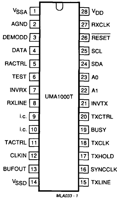
Fig.2 Pinning diagram.
