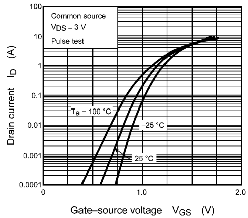
Fig. 7.2 I_D - V_{GS}
