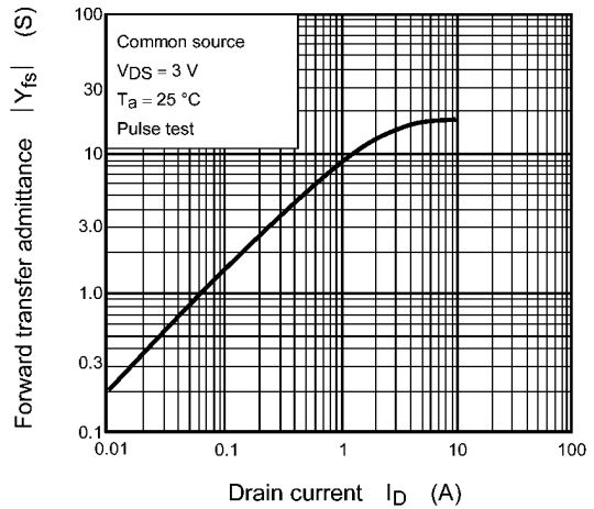
Fig. 7.8 |Y_{fs}| - I_D
