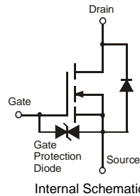
SC-59
