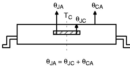
Thermal Resistance — °C/Watt
