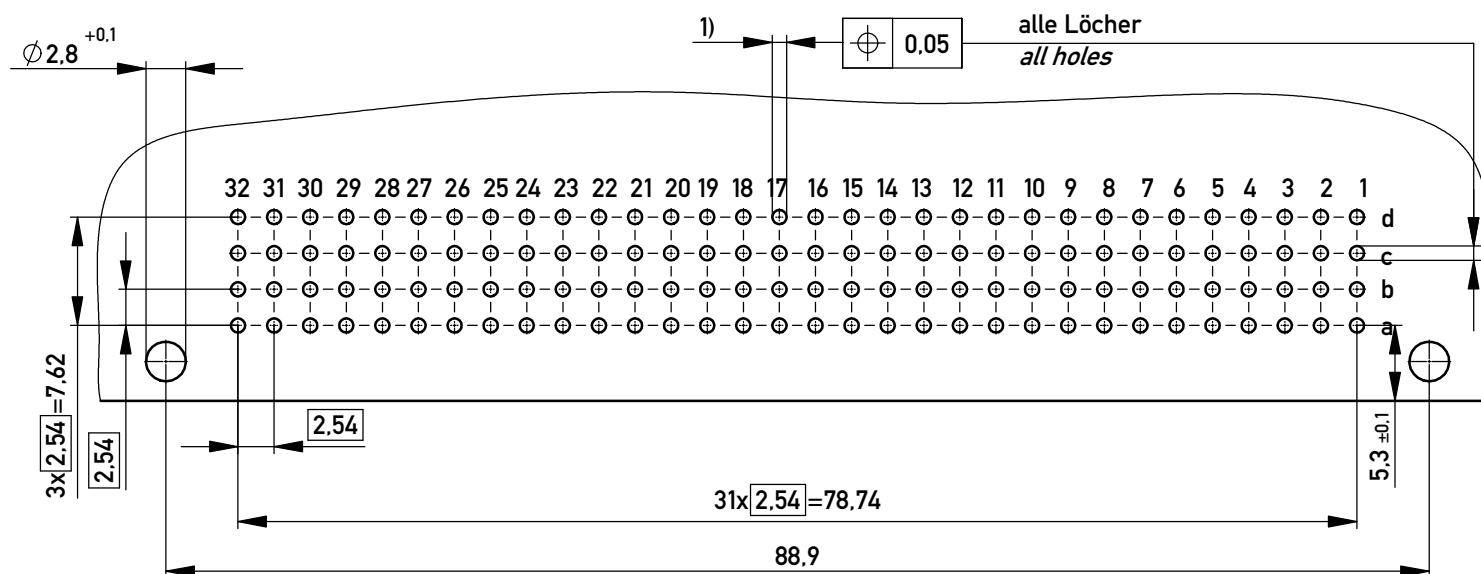
Leiterplatten-Lochbild / PCB drillhole pattern
