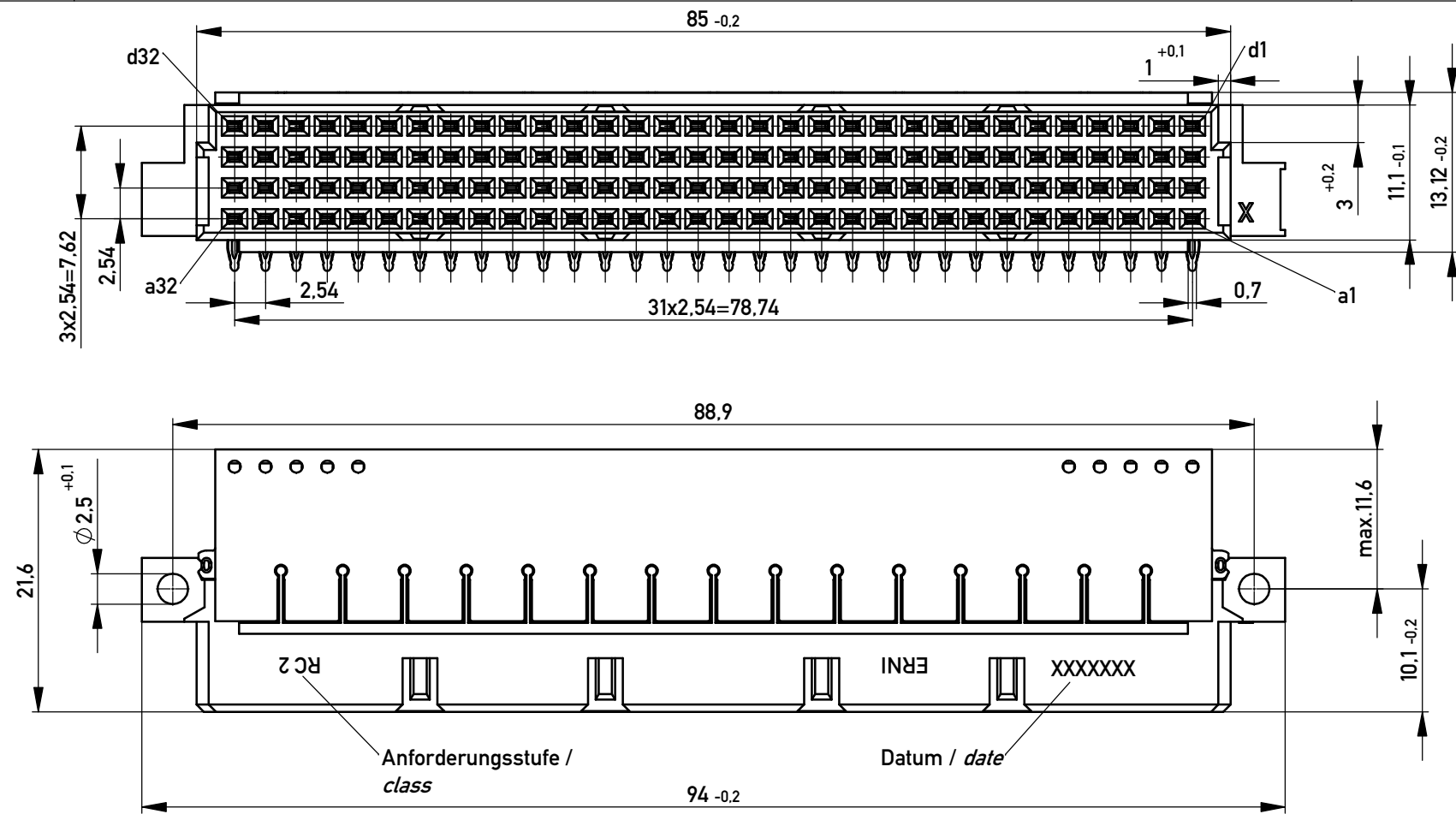
Bestückungsplan / contact layout
