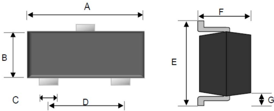
SOT-23
