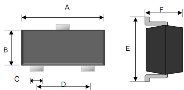
SOT-723
