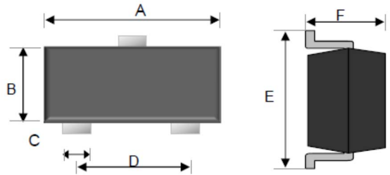
SOT-323
