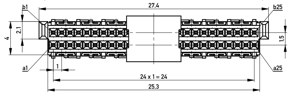
Leiterplatten-Layout Vorschlag / PCB-Layout Proposal
