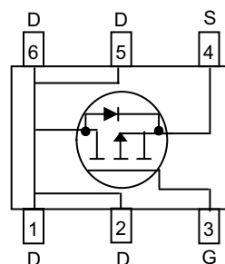
SOT-23-6L
