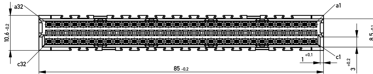
Bestückungsplan / contact layout
