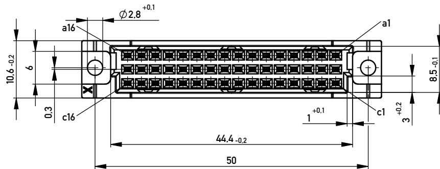
Bestückungsplan / contact layout
