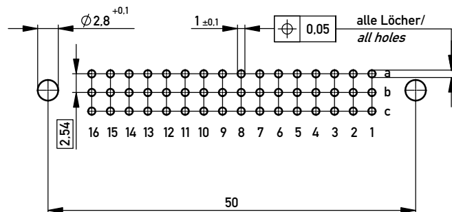
Leiterplatten-Lochbild / PCB drillhole Pattern
