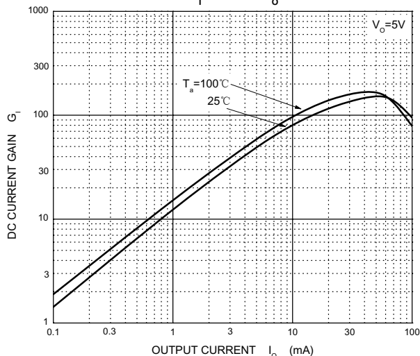
G_i — I_o
