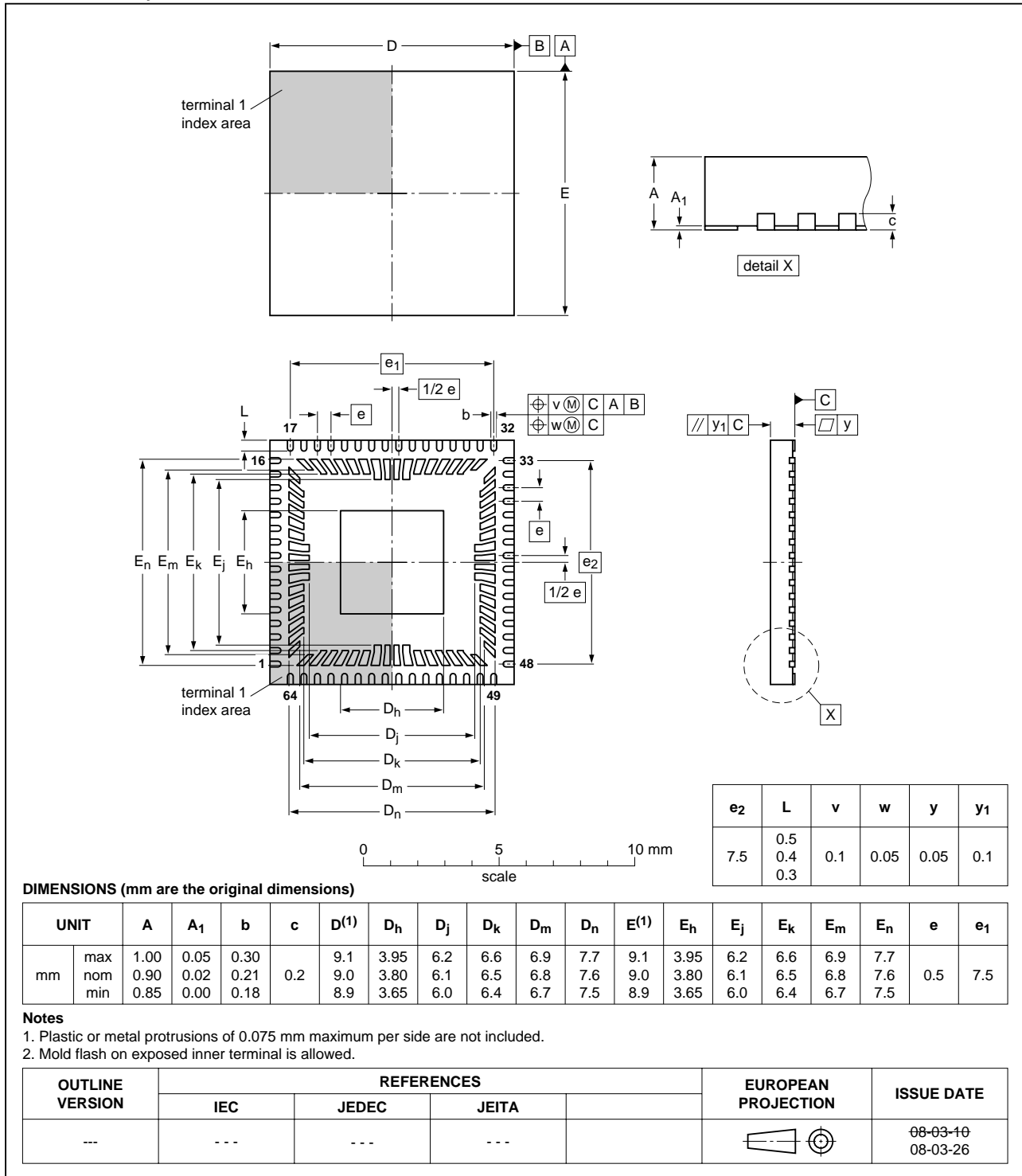
Fig 22. Package outline VFQFPN64
