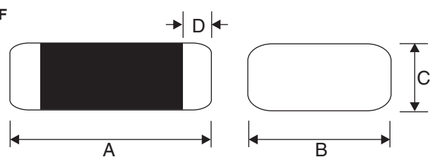
CTCB1812F
