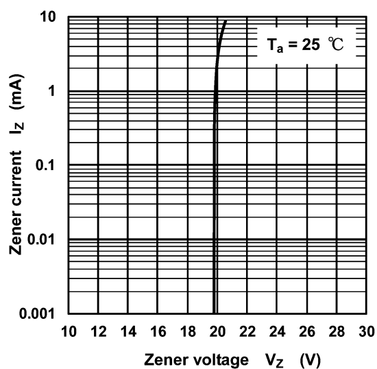
Fig. 8.1 I_Z - V_Z
