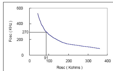
VDD = 5.0V
