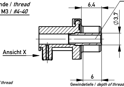
Bolzen / bolt
