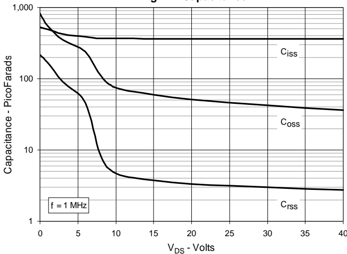
Fig. 11. Capacitance
