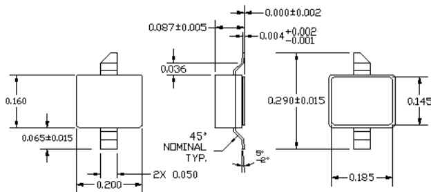
POLYFET S02 PACKAGE
