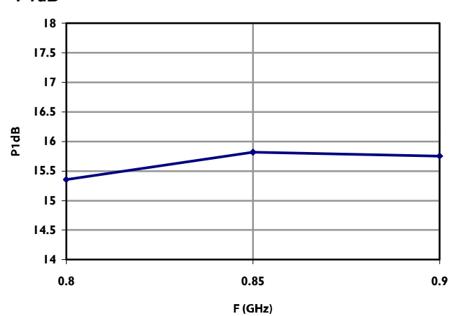
P1dB
