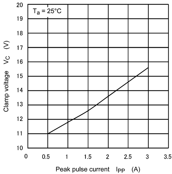
Fig. 9.1 V_C - I_{PP}
