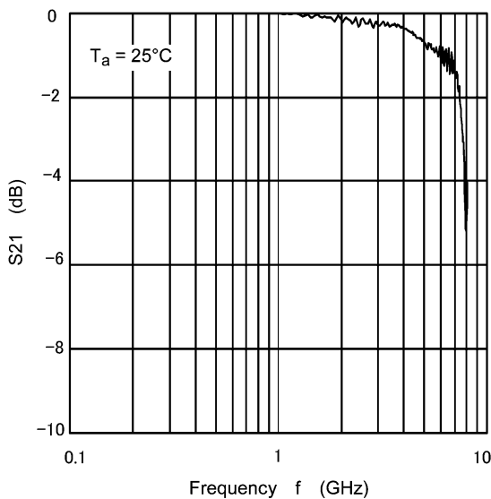
Fig. 10.1 S_{21} - f
