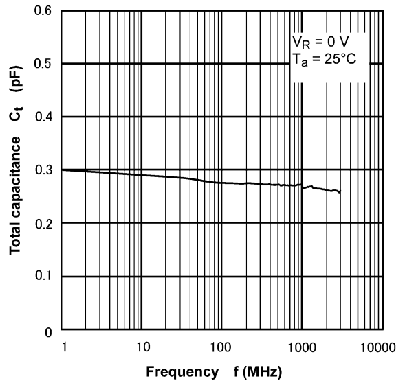
Fig. 8.4 C_t - f
