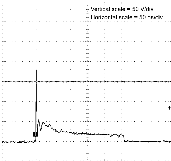
Fig. 11.1 +8 kV
