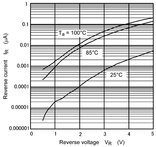
Fig. 8.2 I_R - V_R
