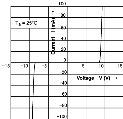
Fig. 8.1 I - V
