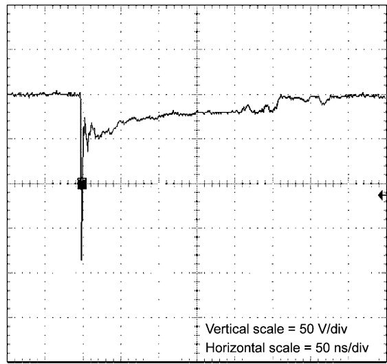
Fig. 11.2 -8 kV
