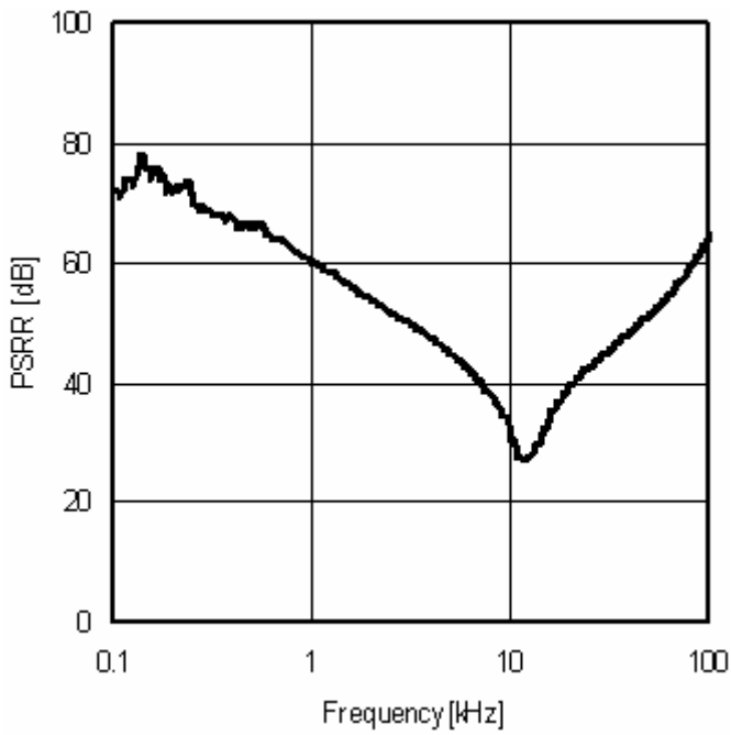
Fig.20 PSRR( I_o=0mA )
