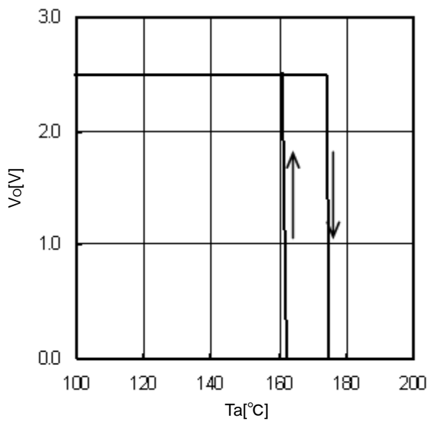
Fig.21 TSD ( I_o=0A )
