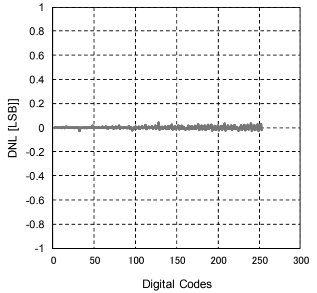
Fig.40 HAVDD DNL
