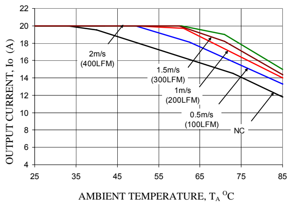
Vo=5.0V
