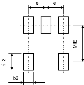
SSOP5
