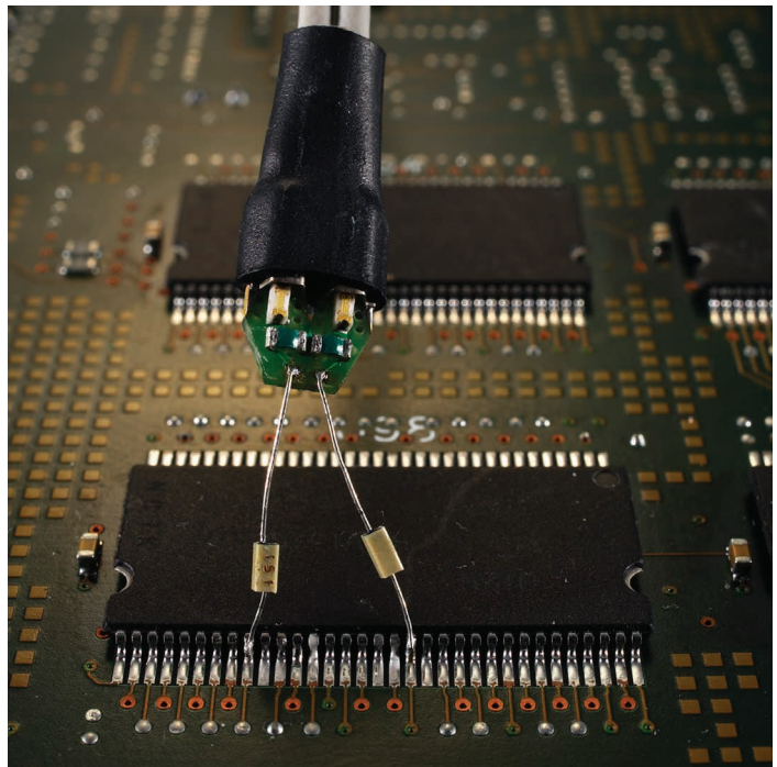
Figure 5. Image using LW ZIF Head
