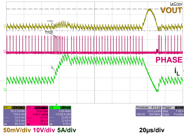
Fig. 16: Load Transient 4-12A
