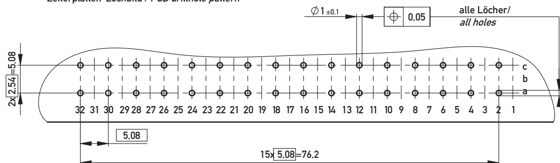
Leiterplatten-Lochbild / PCB drillhole pattern
