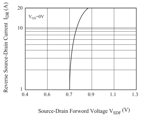
Fig 6. I_{DR} - V_{SDF}
