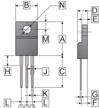
ITO-220
